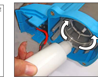
Удалите нагар в цилиндре
